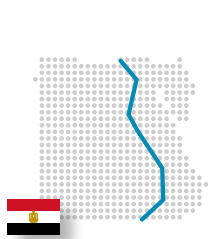
Bacino inferiore del Nilo
