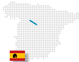
Bacino del Cega
